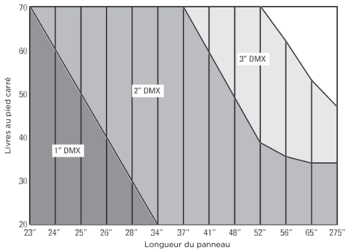
Panneaux de 24" de large 8 mm LTC - 1700 g/m 2
