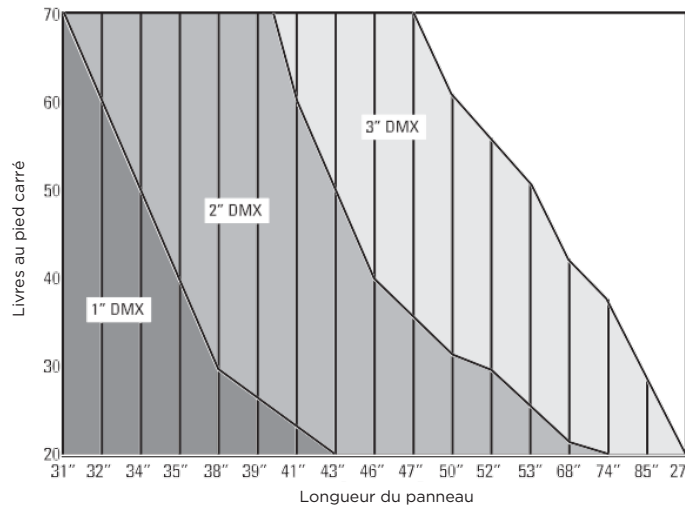
Panneaux de 36" de large 16 mm LTC - 2800 g/m 2
