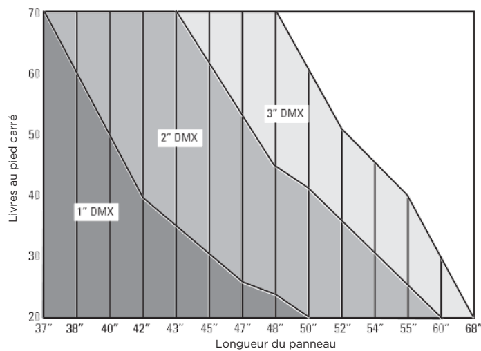
Panneaux de 83" de large 16 mm LTC - 2800 g/m 2
