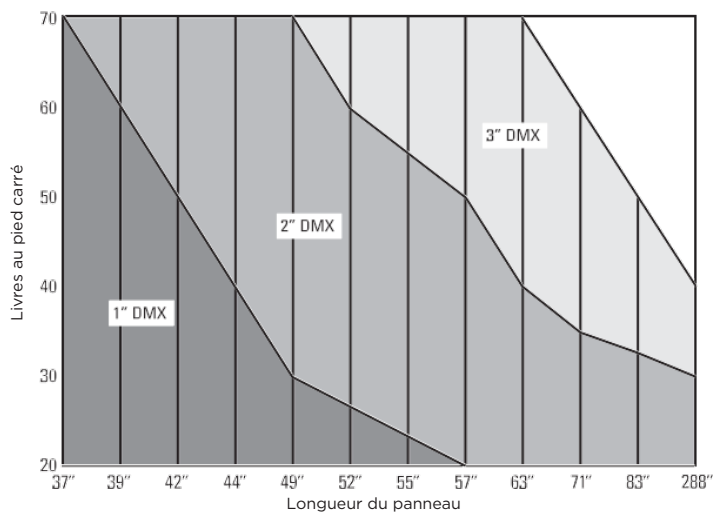
Panneaux de 36" de large 20 mm LTC - 3300 g/m 2
