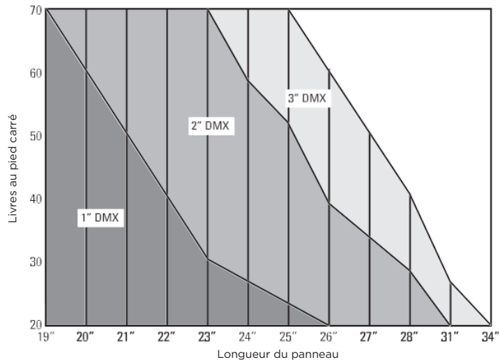
Panneaux de 72" de large 6 mm LTC - 1300 g/m 2
