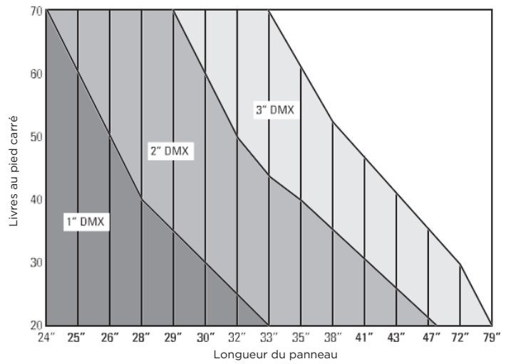
Panneaux de 36" de large 8 mm LTC - 1700 g/m 2
