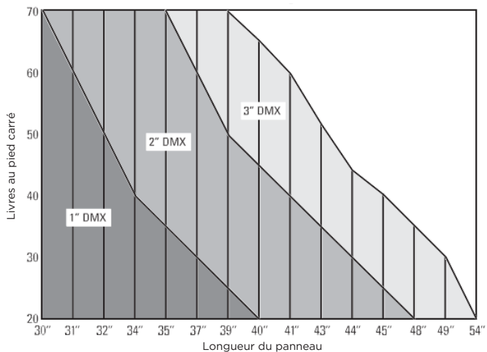
Panneaux de 83" de large 20 mm LTC - 3300 g/m 2
