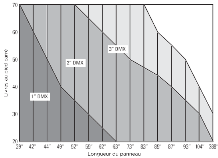
Panneaux de 48" de large 25 mm LTC - 3500 g/m 2
