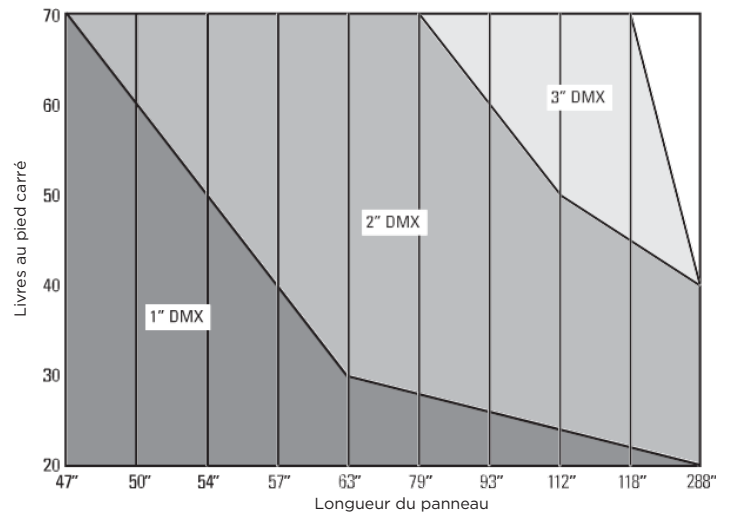
Panneaux de 36" de large 25 mm LTC - 3500 g/m 2
