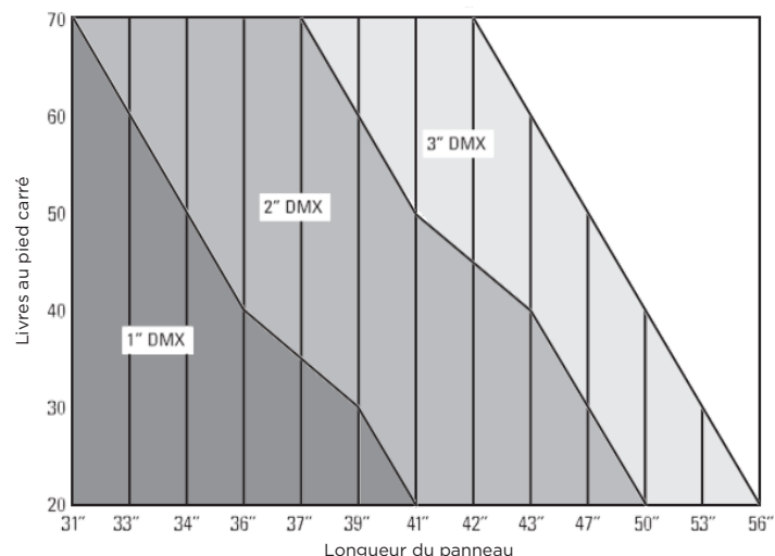
Panneaux de 72" de large 20 mm LTC - 3300 g/m 2
