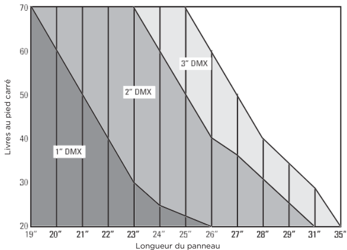
Panneaux de 48" de large 6 mm LTC - 1300 g/m 2
