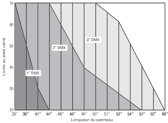
Panneaux de 48" de large 16 mm LTC - 2800 g/m 2
