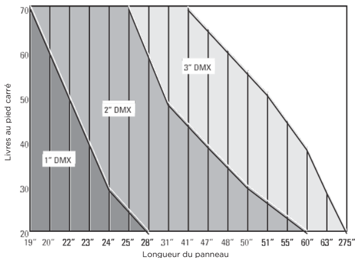
Panneaux de 24" de large 6 mm LTC - 1300 g/m 2
