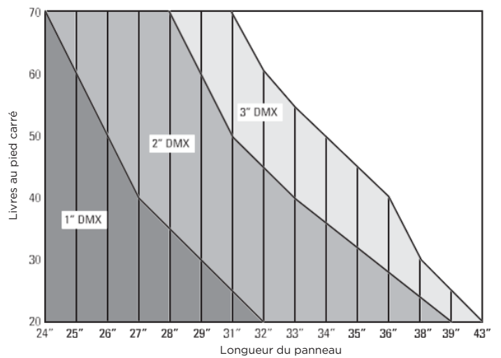
Panneaux de 72" de large 8 mm LTC - 1700 g/m 2
