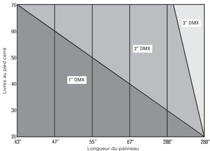
Panneaux de 24" de large 20 mm LTC - 3300 g/m 2
