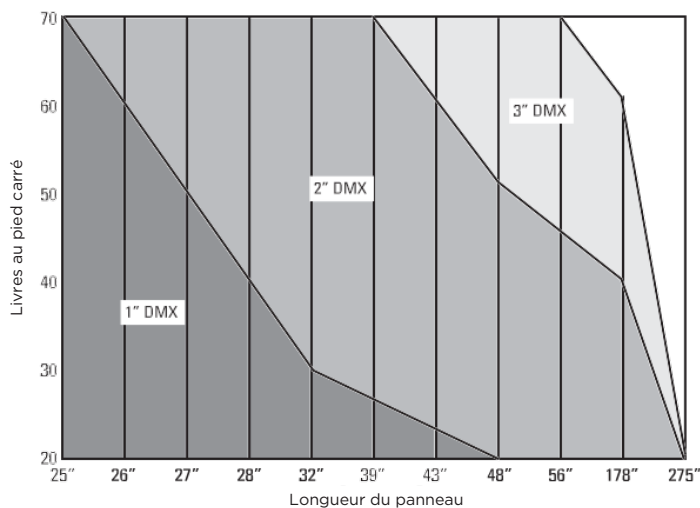
Panneaux de 24" de large 10 mm LTC - 2000 g/m 2
