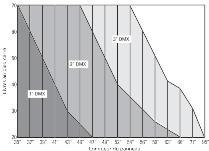
Panneaux de 48" de large 20 mm LTC - 3300 g/m 2
