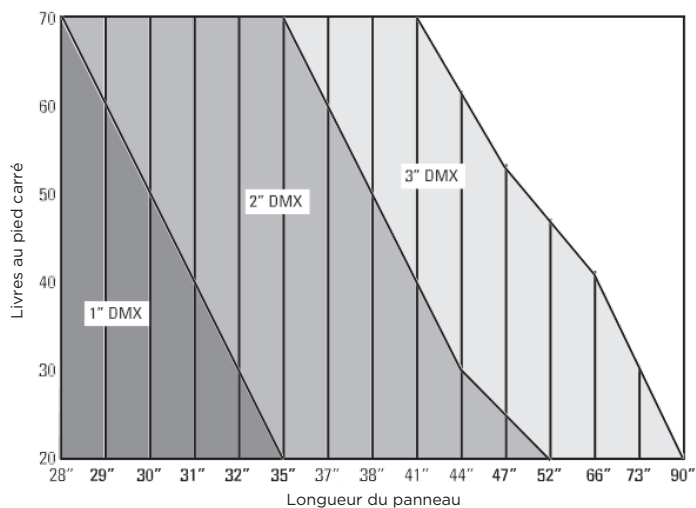
Panneaux de 36" de large 10 mm LTC - 2000 g/m 2
