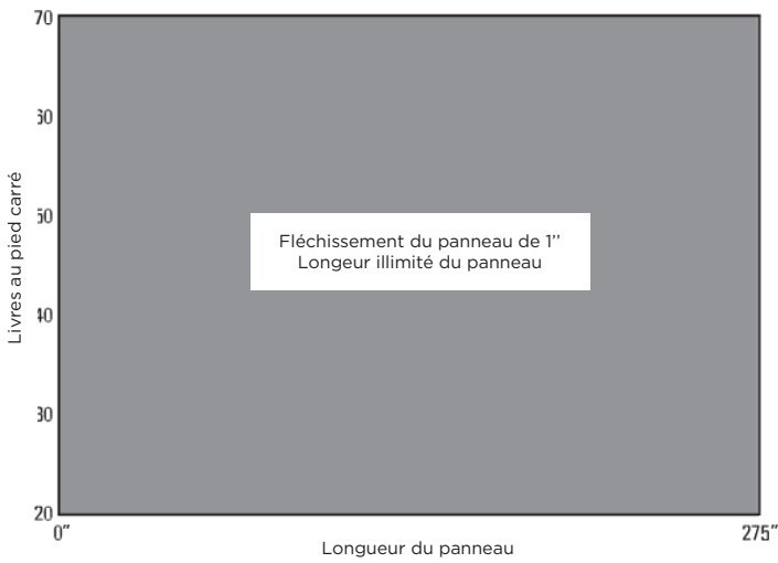
Panneaux de 24" de large 25 mm LTC - 3500 g/m 2
