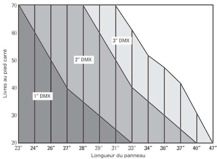
Panneaux de 48" de large 8 mm LTC - 1700 g/m 2
