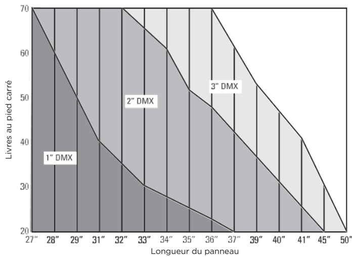
Panneaux de 72" de large 10 mm LTC - 2000 g/m 2
