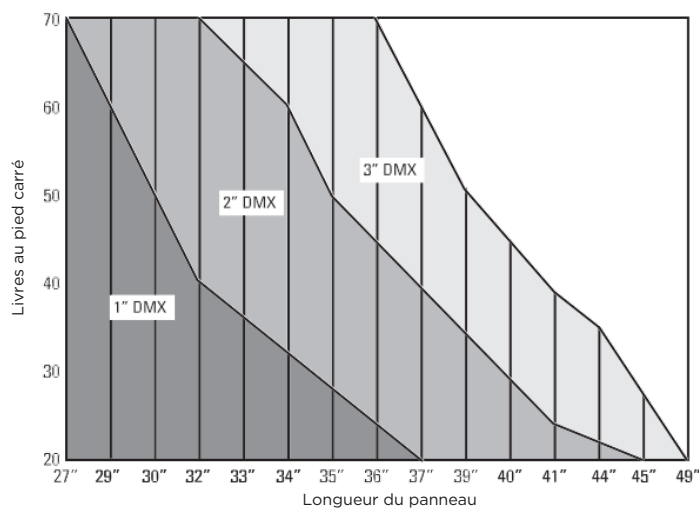
Panneaux de 83" de large 10 mm LTC - 2000 g/m 2
