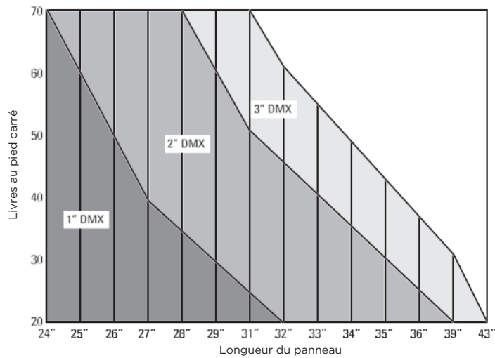
Panneaux de 83" de large 8 mm LTC - 1700 g/m 2
