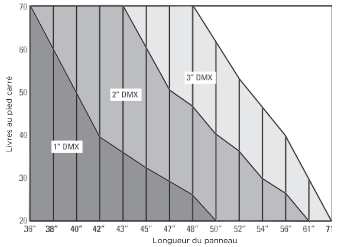
Panneaux de 72" de large 16 mm LTC - 2800 g/m 2
