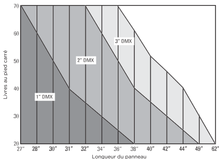
Panneaux de 48" de large 10 mm LTC - 2000 g/m 2
