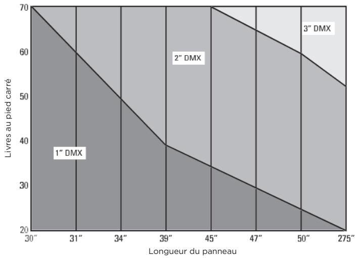
Panneaux de 24" de large 16 mm LTC - 2800 g/m 2
