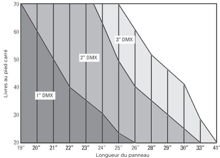
Panneaux de 36" de large 6 mm LTC - 1300 g/m 2
